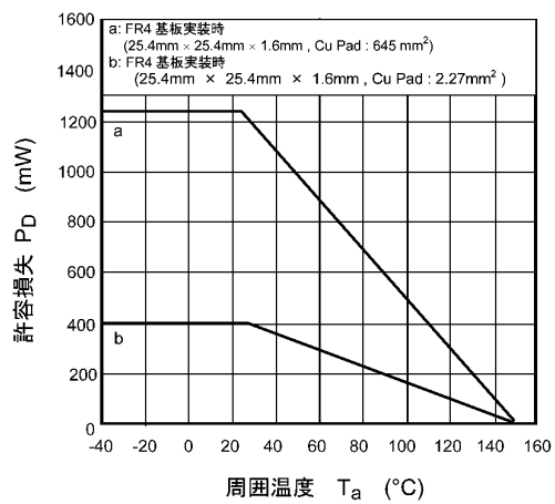
図 8.13 P_D - T_a
