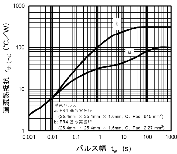
図 8.11 r_{th} - t_w
