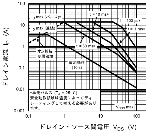
図 8.7 安全動作領域
