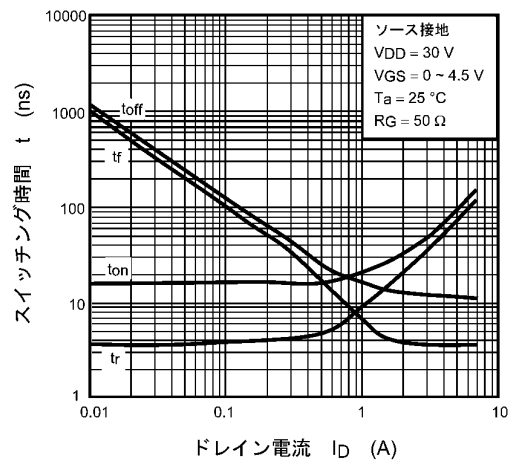
図 8.4 t - I_D
