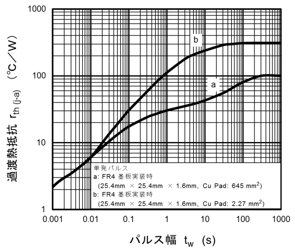
図 8.6 r_{th} - t_w
