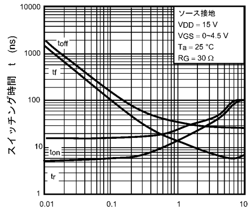
図 8.10 t - I_D
