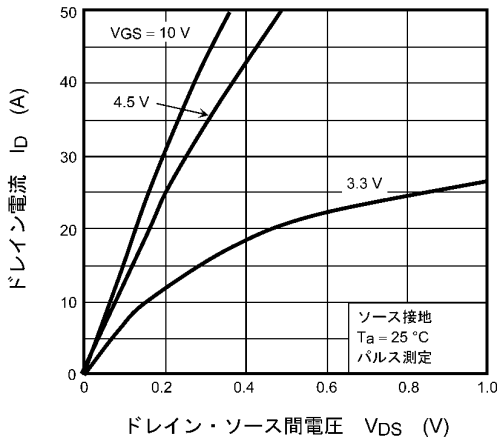
図 8.1 I_D - V_{DS}
