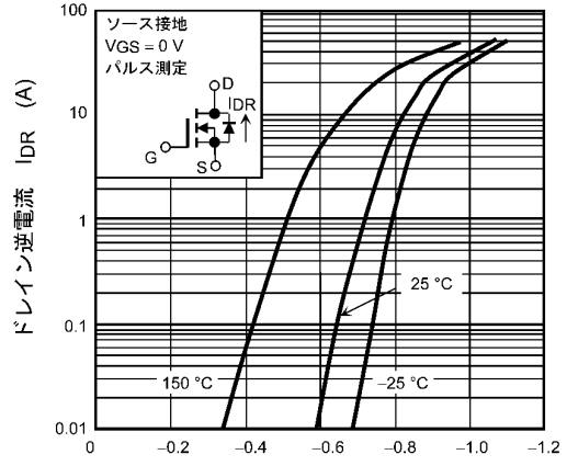
図 8.8 I_{DR} - V_{DS}
