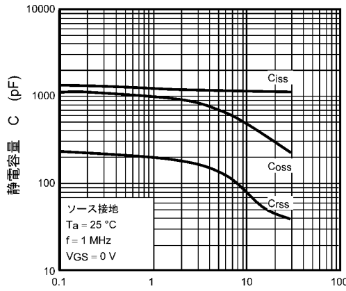
図 8.9 C - V_{DS}
