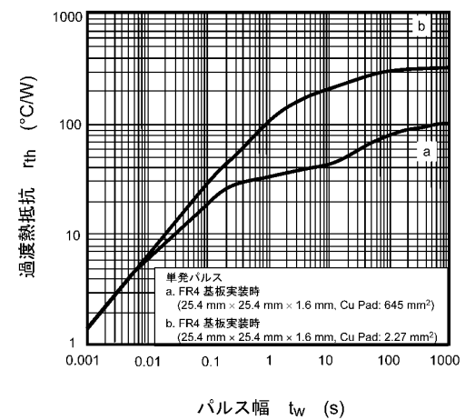
図 8.12 r_{th} - t_w
