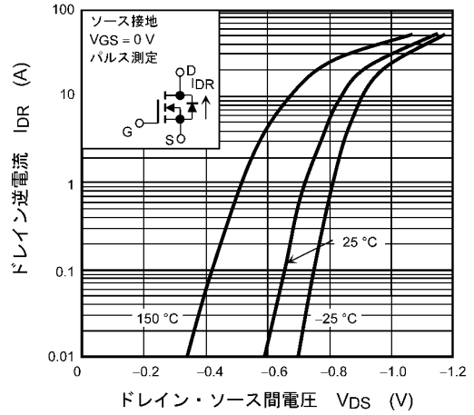
図 8.8 I_{DR} - V_{DS}
