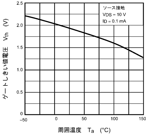
図 8.7 V_{th} - T_a
