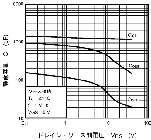
図 8.9 C - V_{DS}
