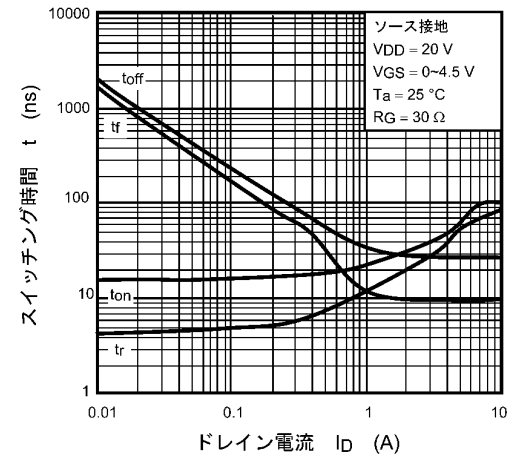
図 8.10 t - I_D
