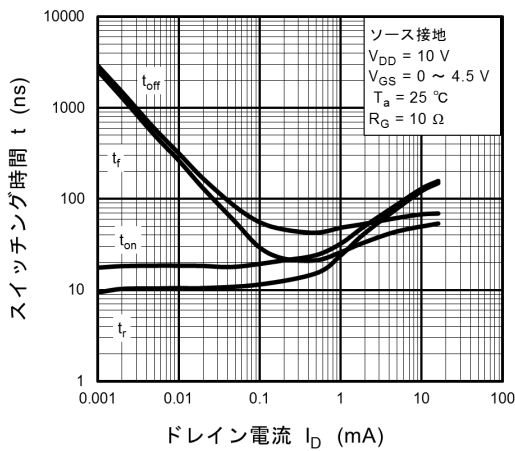
図 8.9 t - I_D
