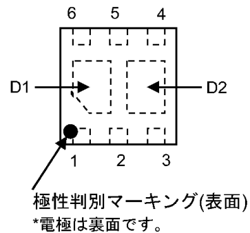
ピン配置(Top View)
