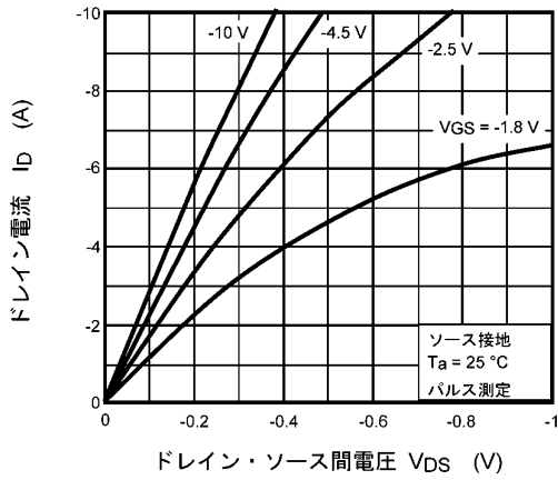
図 7.2.1 I_D - V_{DS}
