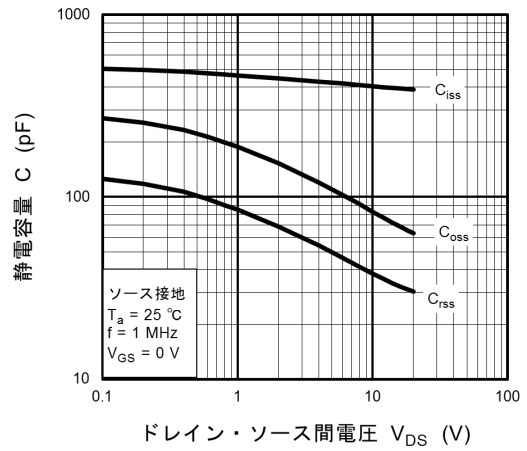
図 7.1.10 C - V_{DS}
