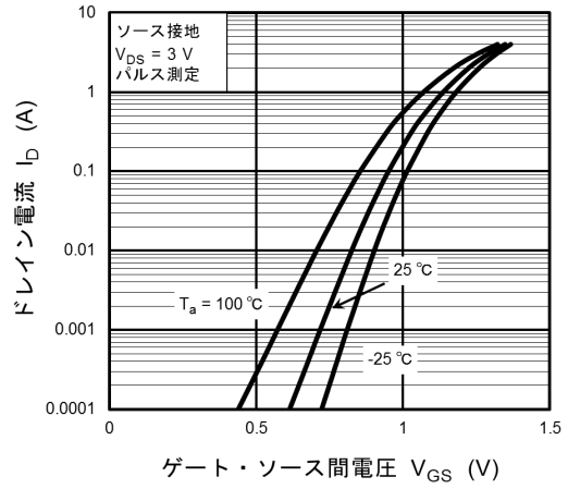
図 7.1.2 I_D - V_{GS}
