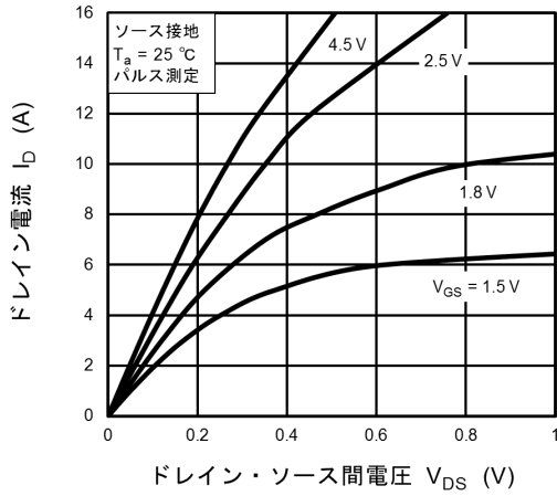
図 7.1.1 I_D - V_{DS}
