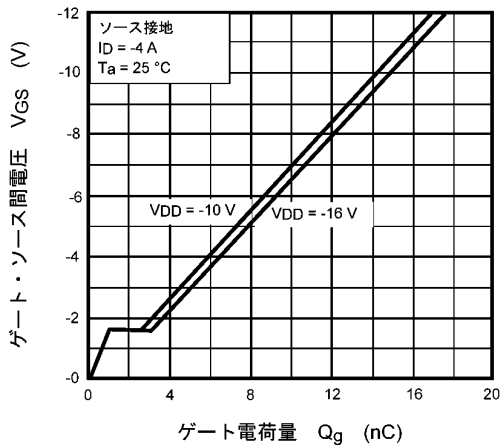
図 7.2.9 ダイナミック入力特性
