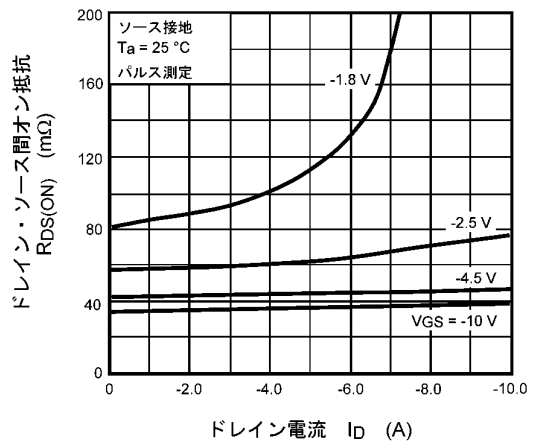
図 7.2.4 R_{DS(ON)} - I_D
