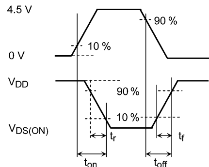
入力波形/出力波形
