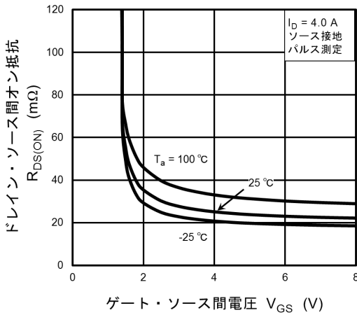
図 7.1.3 R_{DS(ON)} - V_{GS}
