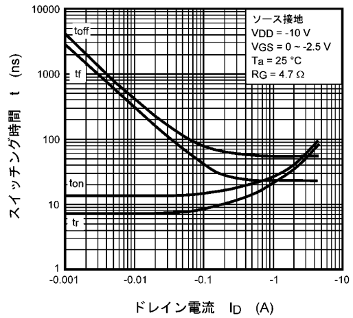
図 7.2.8 t - I_D
