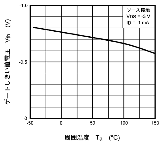
図 7.2.6 V_{th} - T_a
