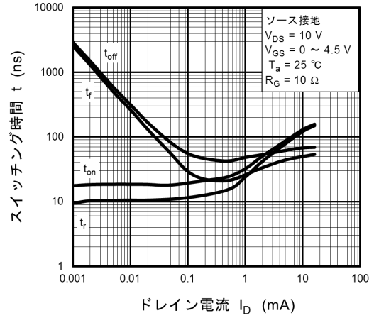
図 7.1.8 t - I_D
