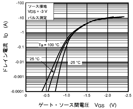
図 7.2.2 I_D - V_{GS}
