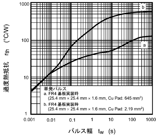
図 7.3.1 r_{th} - t_w
