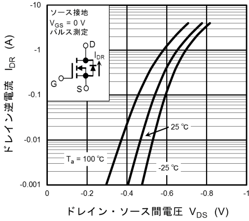
図 7.1.7 I_{DR} - V_{DS}
