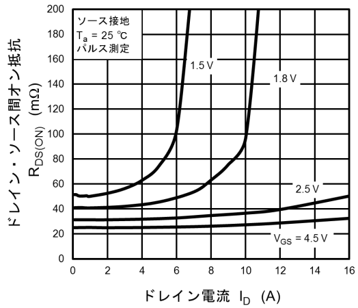
図 7.1.4 R_{DS(ON)} - I_D
