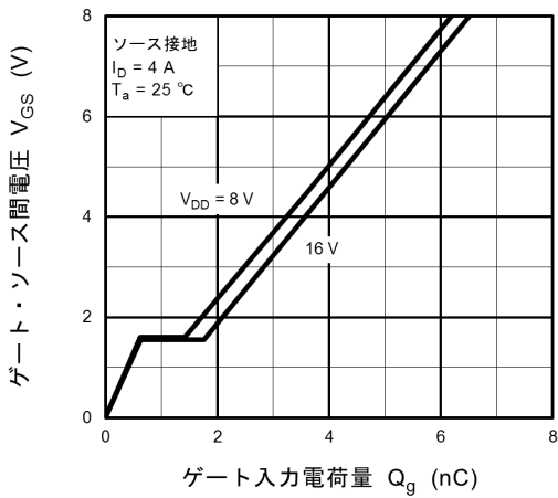
図 7.1.9 ダイナミック入力特性
