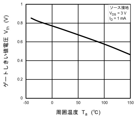
図 7.1.6 V_{th} - T_a
