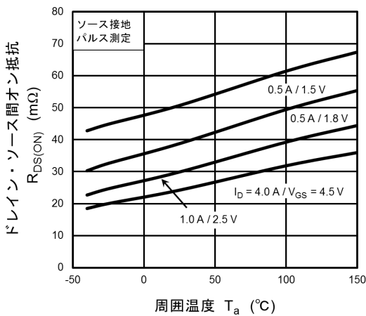
図 7.1.5 R_{DS(ON)} - T_a
