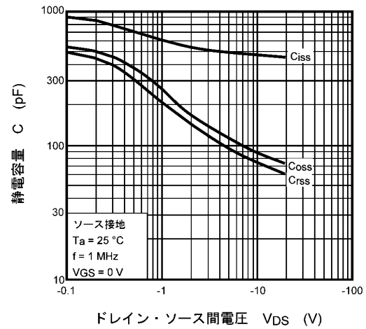
図 7.2.10 C - V_{DS}
