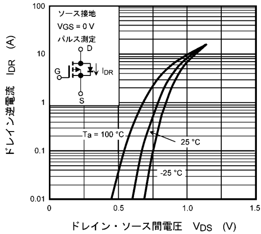
図 7.2.7 I_{DR} - V_{DS}
