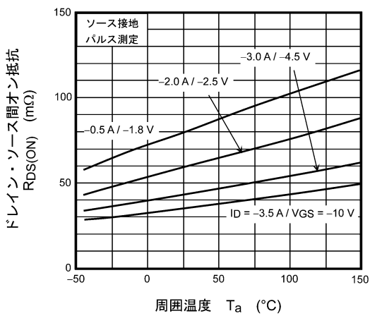
図 7.2.5 R_{DS(ON)} - T_a
