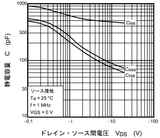
図 7.2.8 C - V DS
