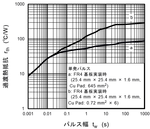
図 7.3.1 r_{th} - t_w
