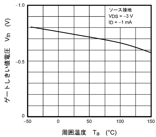
図 7.2.6 V_{th} - T_a
