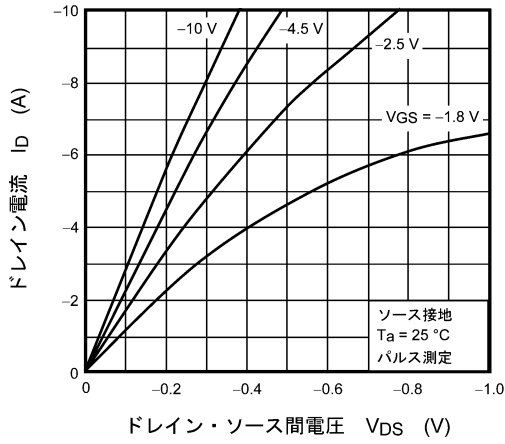
図 7.2.1 I_D - V_{DS}
