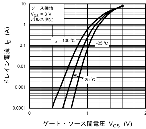
図 7.1.2 I_D - V_{GS}
