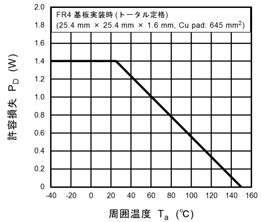
図 7.3.2 P_D - T_a
