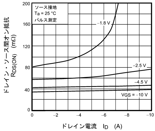
図 7.2.4 R_{DS(ON)} - I_D
