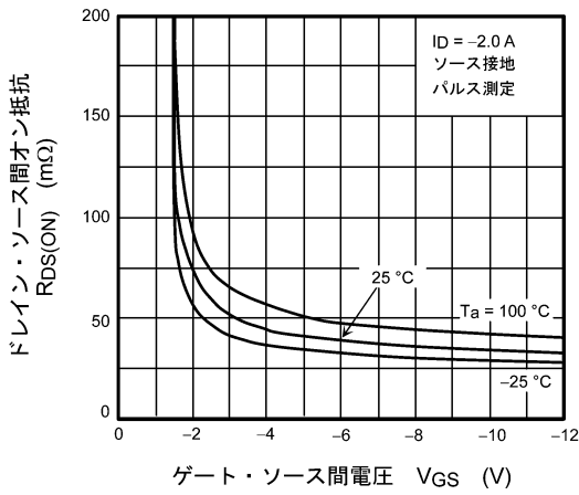
図 7.2.3 R_{DS(ON)} - V_{GS}
