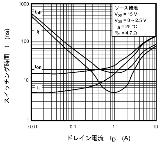
図 7.1.10 t - I_D
