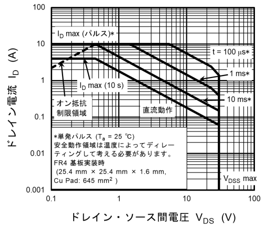
図 7.1.12 安全動作領域
