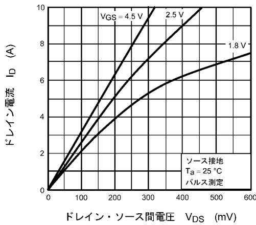
図 7.1.1 I_D - V_{DS}
