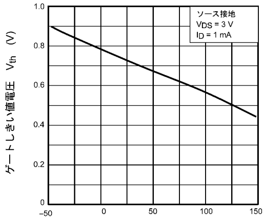
図 7.1.7 V_{th} - T_a
