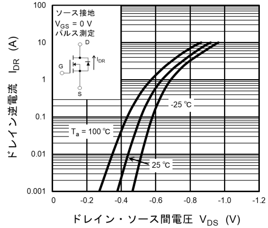
図 7.1.8 I_{DR} - V_{DS}
