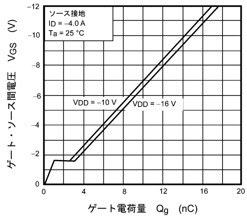
図 7.2.10 ダイナミック入力特性
