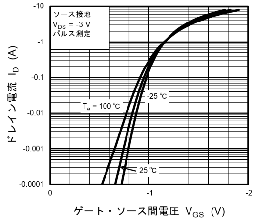
図 7.2.2 I_D - V_{GS}
