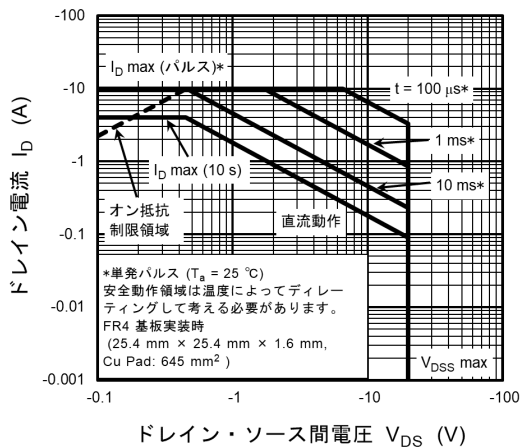
図 7.2.11 安全動作領域
