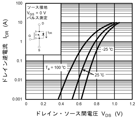
図 7.2.7 I DR - V DS
