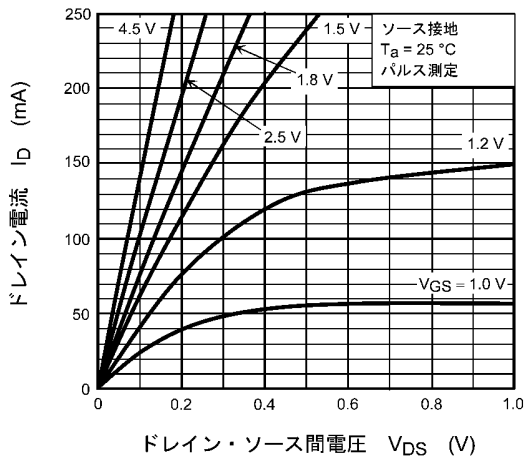
図 7.1 I_D - V_{DS}
