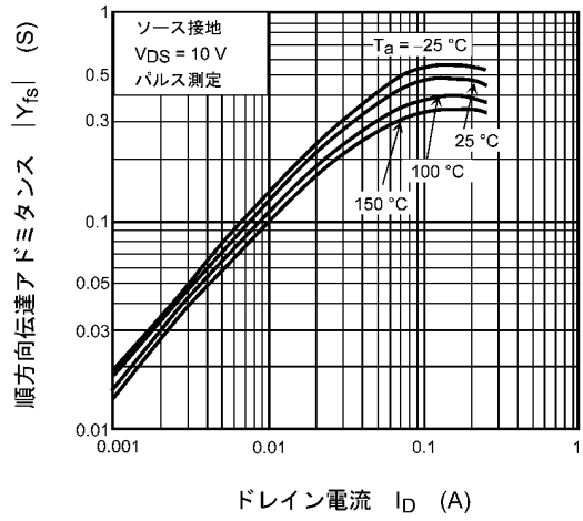
図 7.8 |Y_{fs}| - I_D
