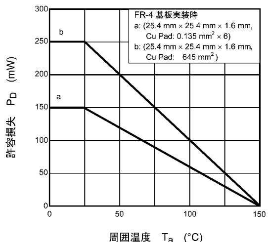
図 7.13 P_D - T_a
