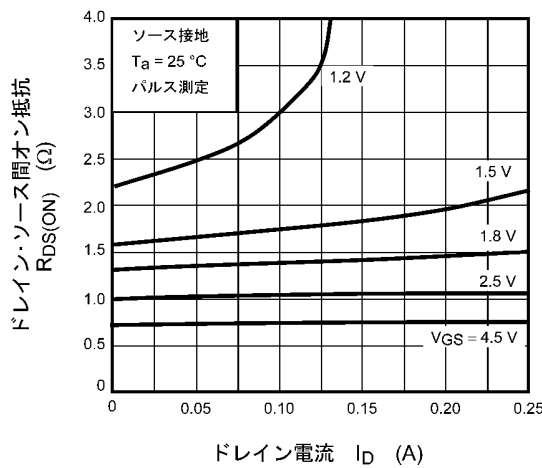
図 7.5 R_{DS(ON)} - I_D
