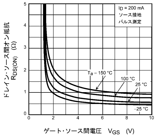
図 7.4 R_{DS(ON)} - V_{GS}
