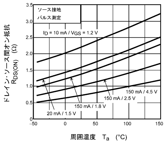
図 7.6 R_{DS(ON)} - T_a
