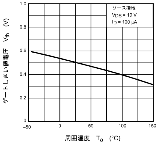
図 7.7 V_{th} - T_a
