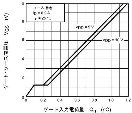
図 7.12 ダイナミック入力特性
