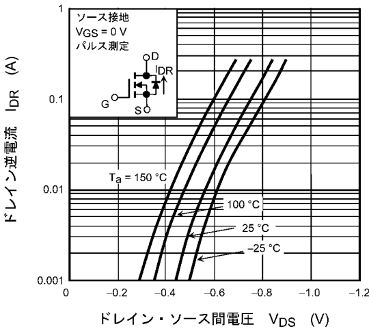
図 7.9 I_{DR} - V_{DS}
