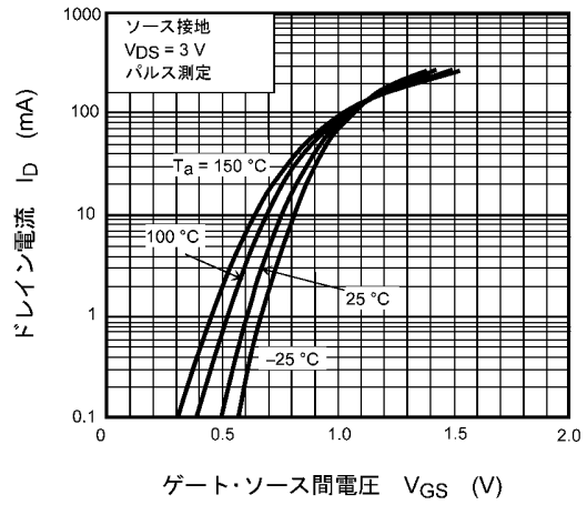
図 7.2 I_D - V_{GS}
