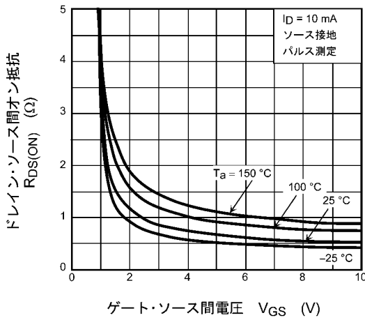
図 7.3 R_{DS(ON)} - V_{GS}
