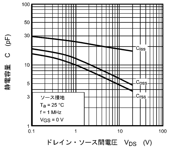
図 7.10 C - V_{DS}
