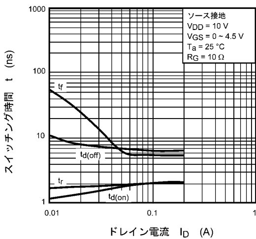
図 7.11 t - I_D
