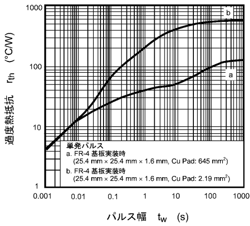
図 7.13 r_{th} - t_w
