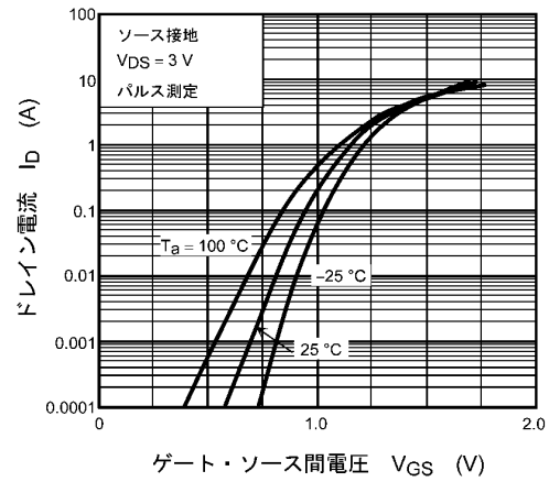
図 7.2 I_D - V_{GS}
