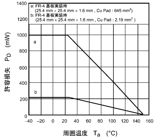
図 7.14 P_D - T_a
