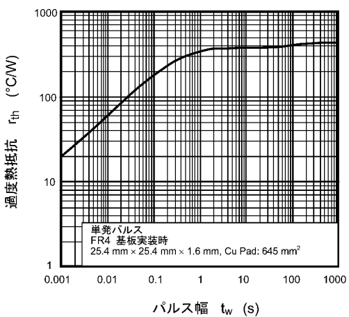
図 8.11 r_{th} - t_w
