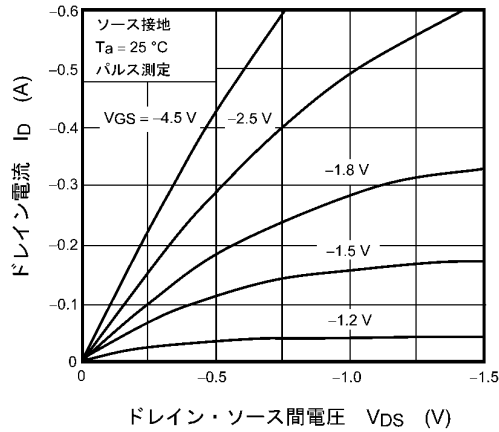
図 8.1 I_D - V_{DS}
