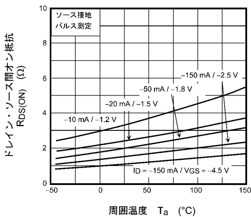
図 8.5 R_{DS(ON)} - T_a
