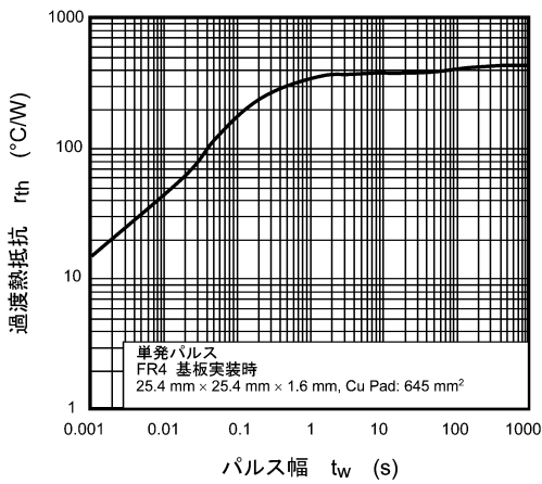
図 8.11 r_{th} - t_w
