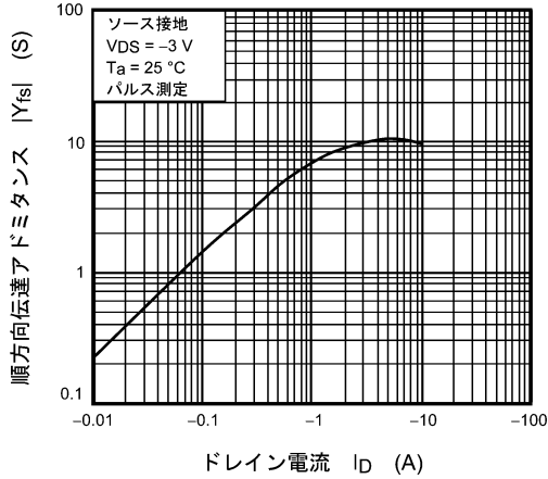
図 8.7 |Y_{fs}| - I_D
