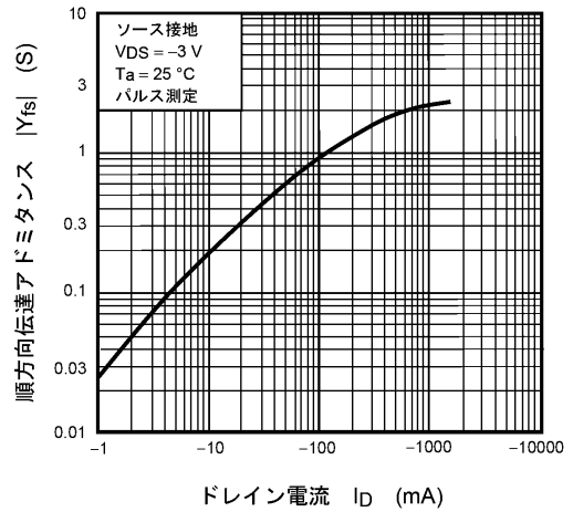
図 7.8 |Y_{fs}| - I_D
