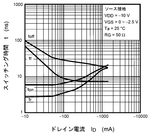
図 7.11 t - I_D
