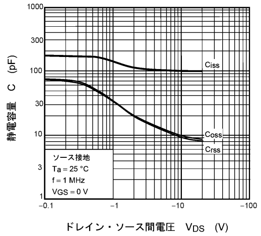
図 7.10 C - V_{DS}
