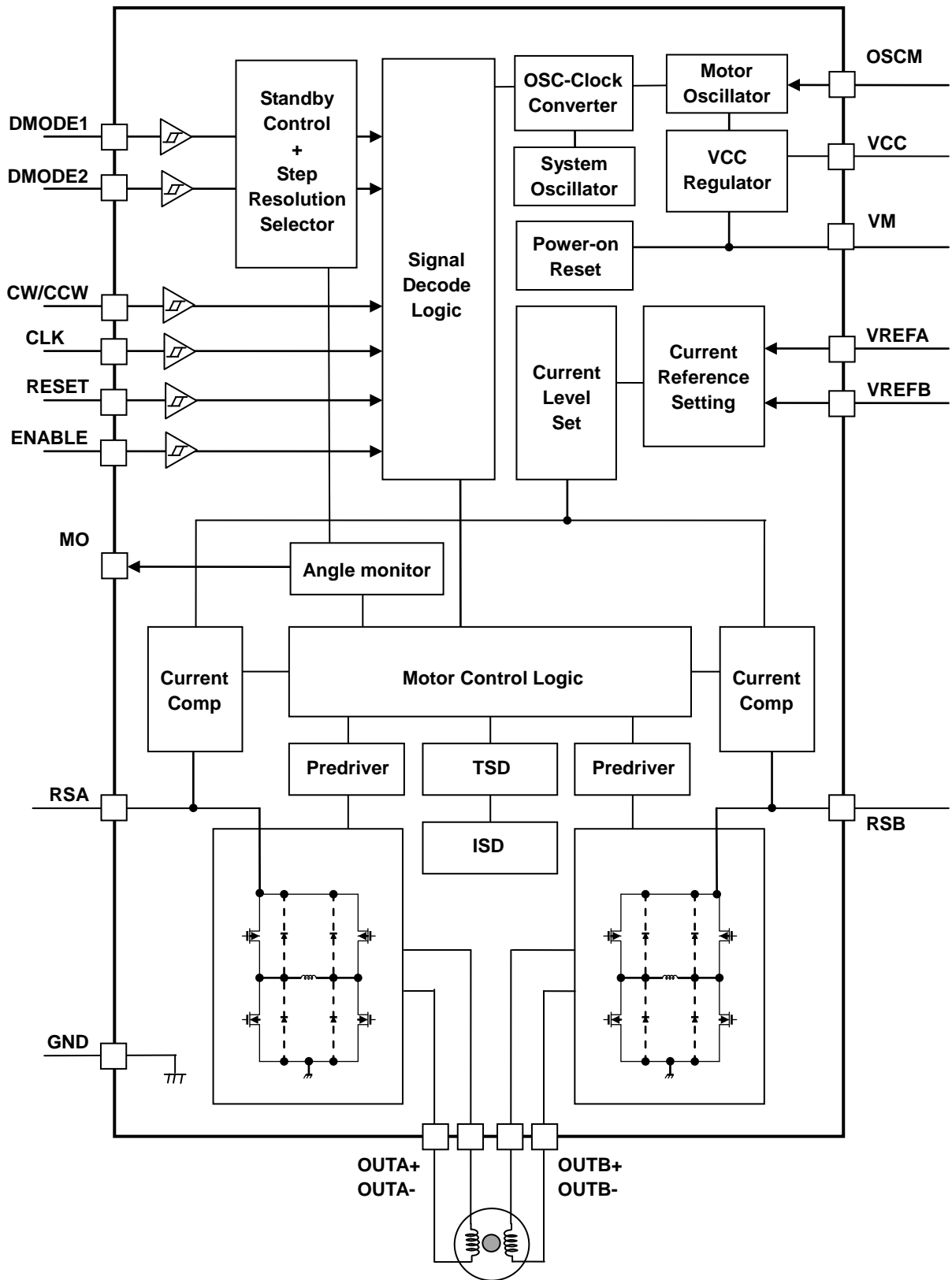
TB62215A ブロック図
