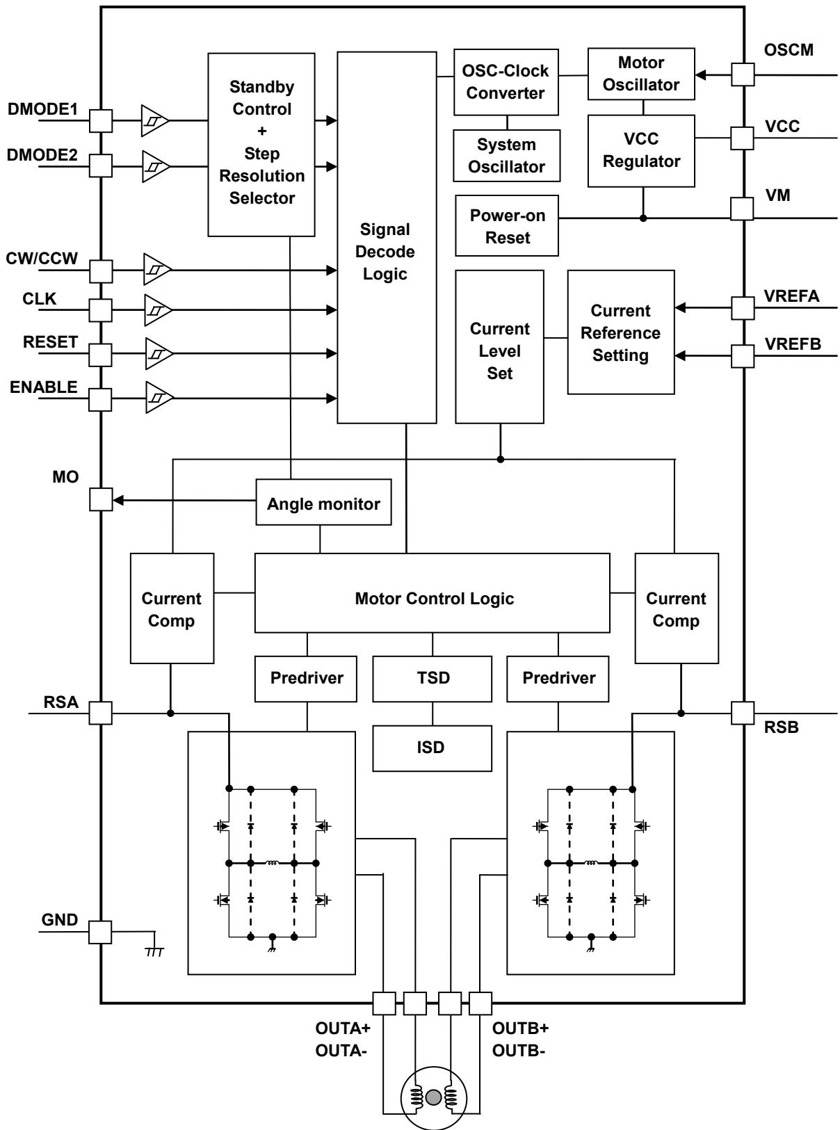
TB67S102A ブロック図
