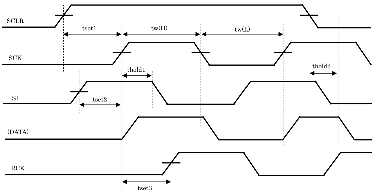
出カトランジスタ・スイッチング特性のタイミング
