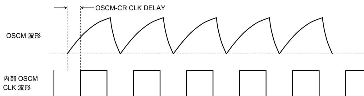
図 2 タイミング波形と名称 (OSCMと内部信号出力)
