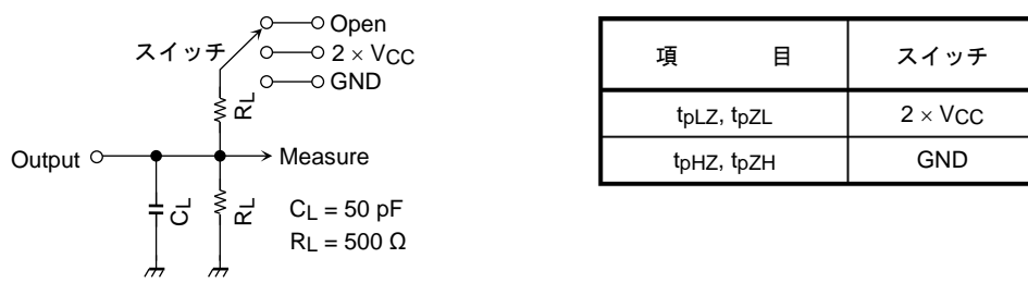
図 1 AC 特性測定回路
