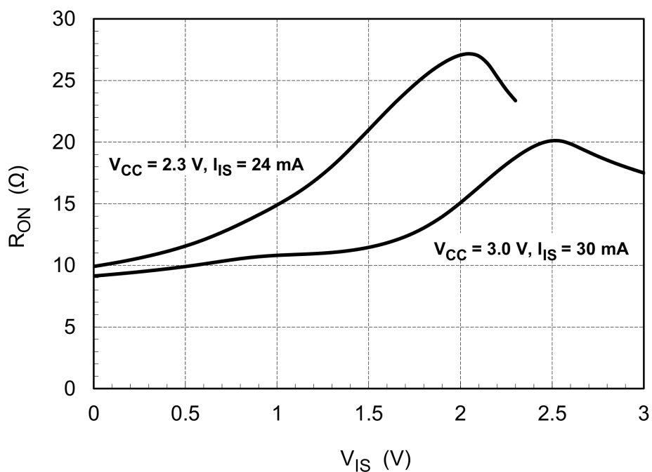
図 13.1 R_{ON} - V_{IS} ( T_a = 25^\circ\text{C} )
