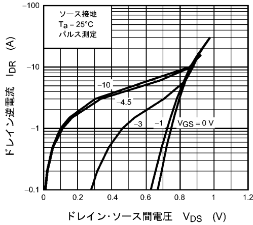
図 8.7 I_{DR} - V_{DS}
