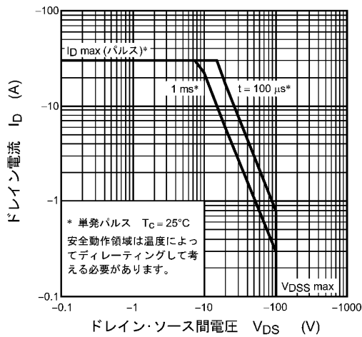
図 8.13 安全動作領域 (最大値 (保証値))
