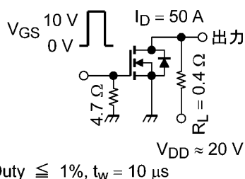
図 6.2.1 スwitchング時間の測定回路
