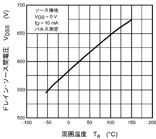
図 8.5 V_{DSS} - T_a
