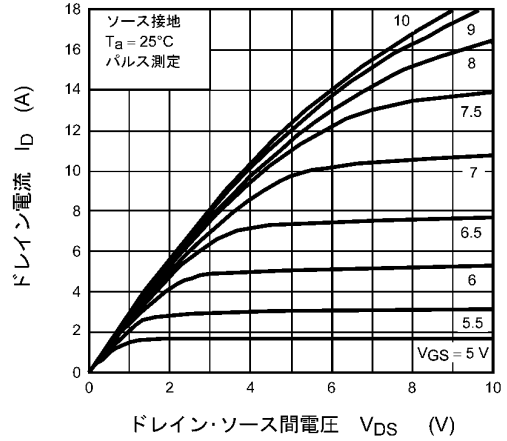
図 8.2 I_D - V_{DS}
