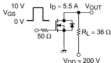
Duty \leq 1\% , t_w = 10\ \mu\text{s} 図 6.2.1 スwitching時間の測定回路例
