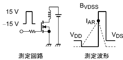
測定回路
