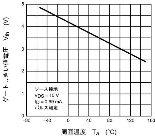
図 8.11 V_{th} - T_a
