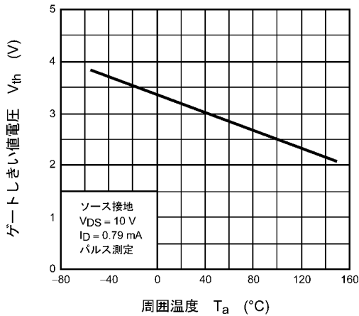
図 8.11 V_{th} - T_a
