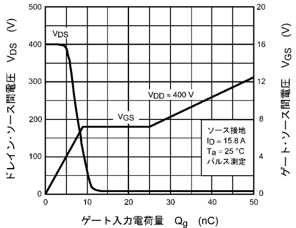
図 8.12 ダイナミック入出力特性
