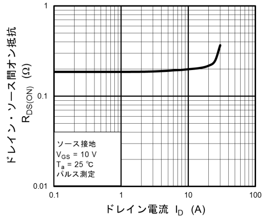
図 8.6 R_{DS(ON)} - I_D
