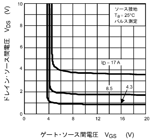
図 8.4 V_{DS} - V_{GS}
