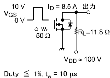
図 6.2.1 スwitching時間の測定回路例
