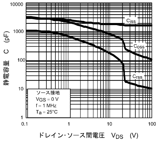
図 8.9 C - V_{DS}
