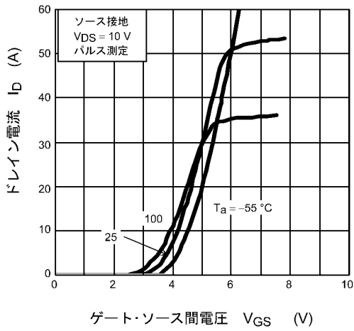
図 8.3 I_D - V_{GS}
