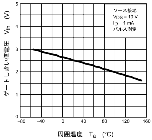
図 8.10 V_{th} - T_a
