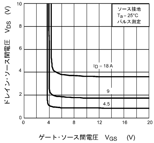
図 8.4 V_{DS} - V_{GS}
