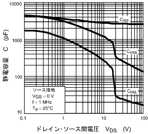
図 8.9 C - V_{DS}
