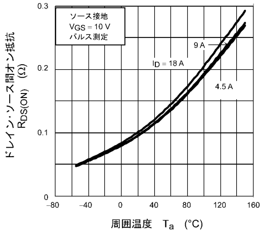
図 8.7 R_{DS(ON)} - T_a
