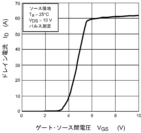
図 8.3 I_D - V_{GS}
