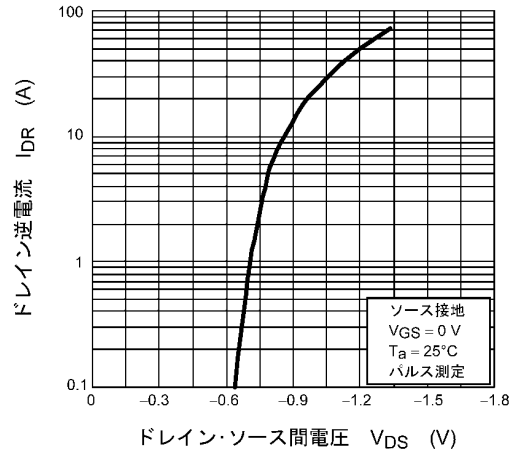
図 8.8 I_{DR} - V_{DS}
