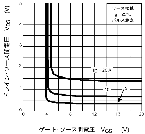
図 8.4 V_{DS} - V_{GS}
