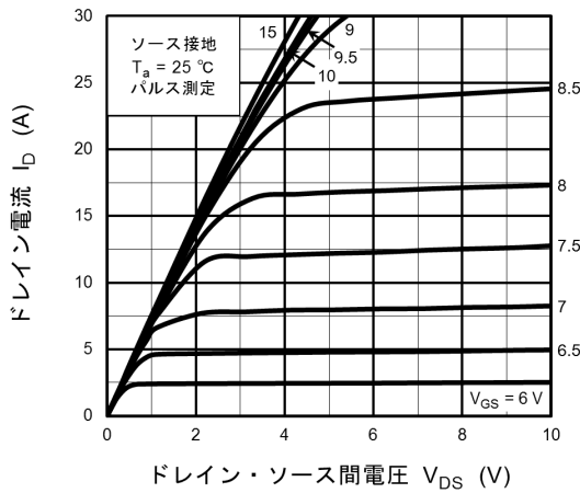
図 8.1 I_D - V_{DS}
