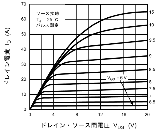
図 8.2 I_D - V_{DS}
