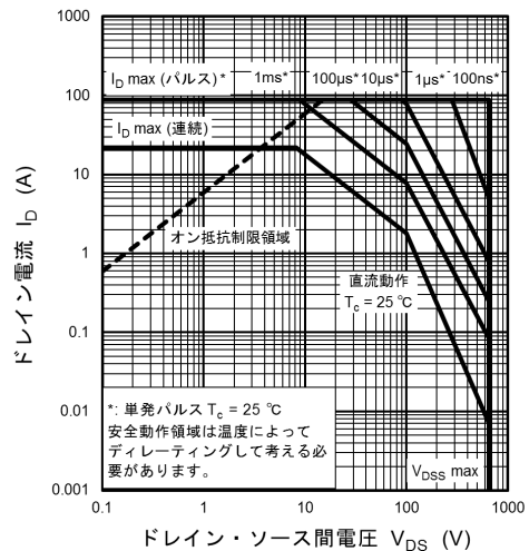
図 8.17 安全動作領域 (最大値 (保証値))
