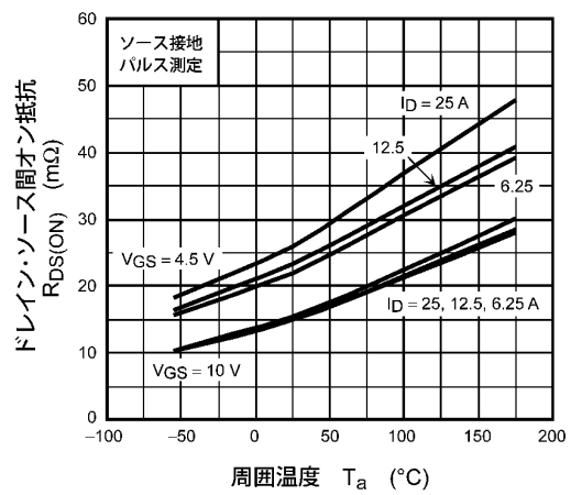
図 8.6 R_{DS(ON)} - T_a
