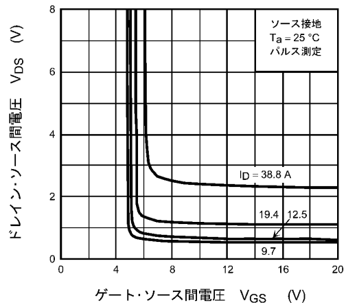
図 8.4 V_{DS} - V_{GS}
