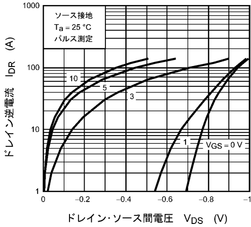
図 8.7 I_{DR} - V_{DS}
