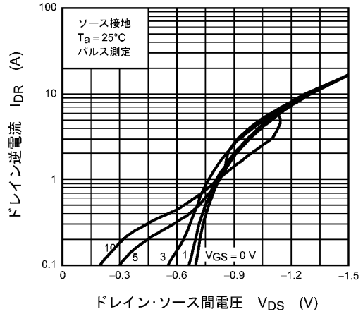
図 8.8 I_{DR} - V_{DS}
