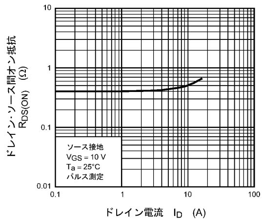
図 8.6 R_{DS(\text{ON})} - I_D
