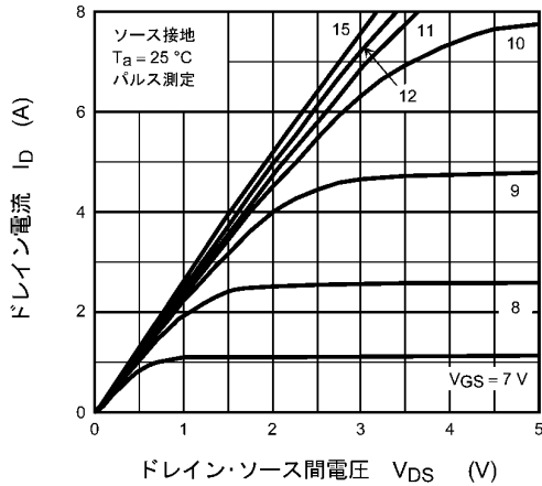
図 8.1 I_D - V_{DS}
