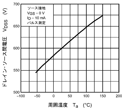
図 8.5 V_{DSS} - T_a
