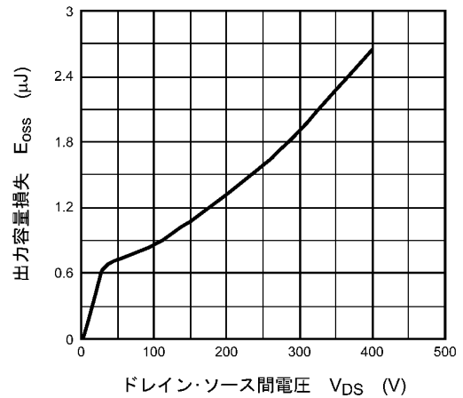
図 8.10 E_{oss} - V_{DS}
