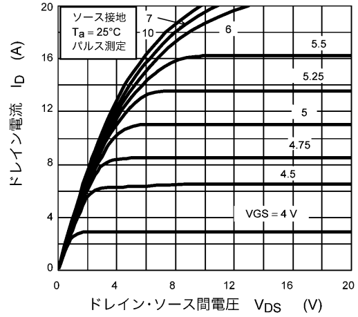
図 8.2 I_D - V_{DS}
