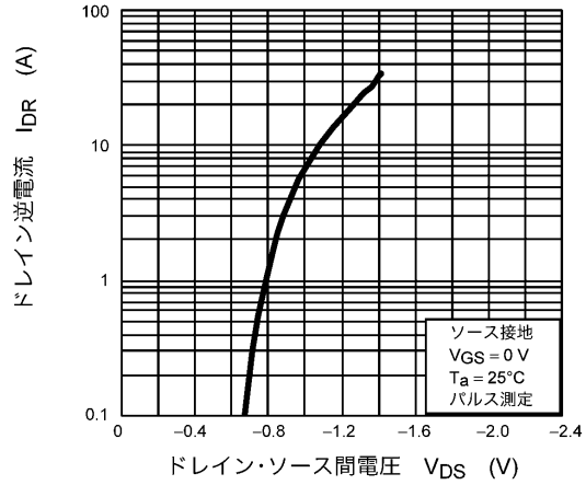
図 8.8 I_{DR} - V_{DS}
