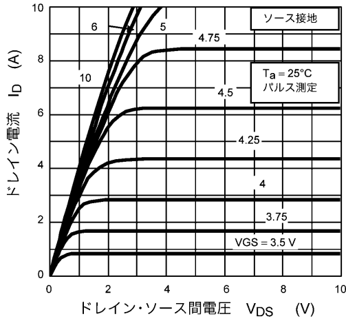
図 8.1 I_D - V_{DS}
