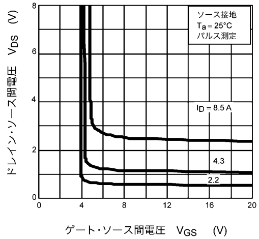
図 8.4 V_{DS} - V_{GS}
