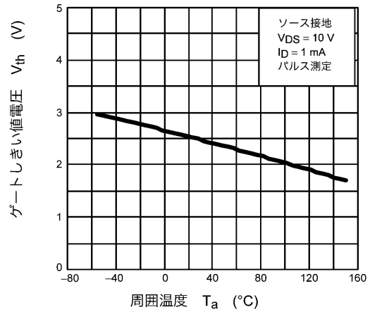
図 8.10 V_{th} - T_a
