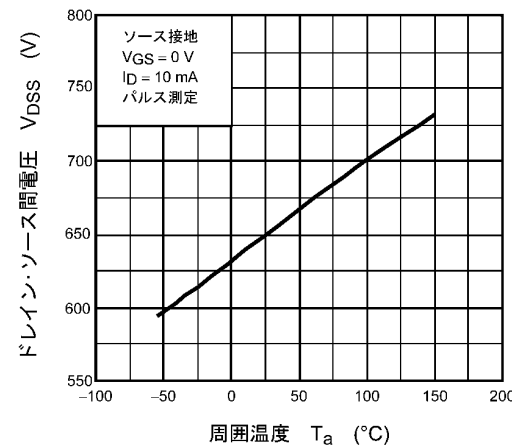
図 8.5 V_{DS} - T_a
