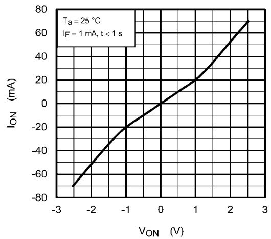
図 12.1.4 I_{ON} - V_{ON}
