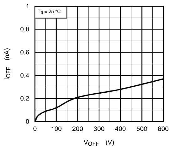
図 12.1.10 I_{OFF} - V_{OFF}
