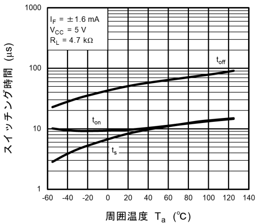
図 11.17 スwitchング時間 - T_a
