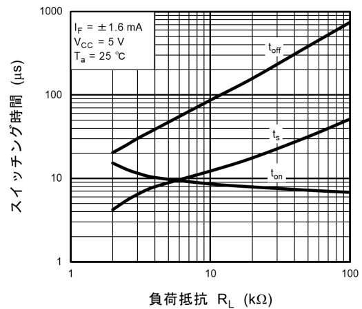
図 11.16 スwitchング時間 - R_L
