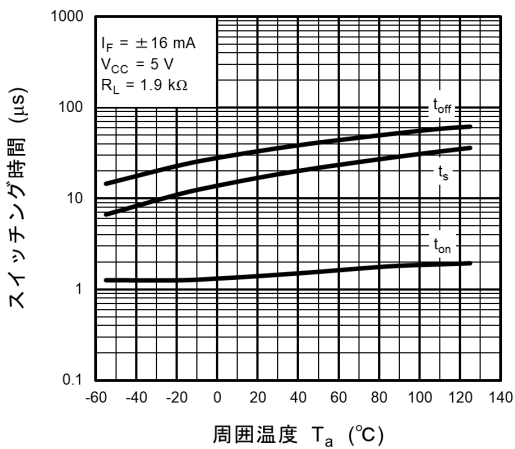
図 11.15 スwitchング時間 - T_a
