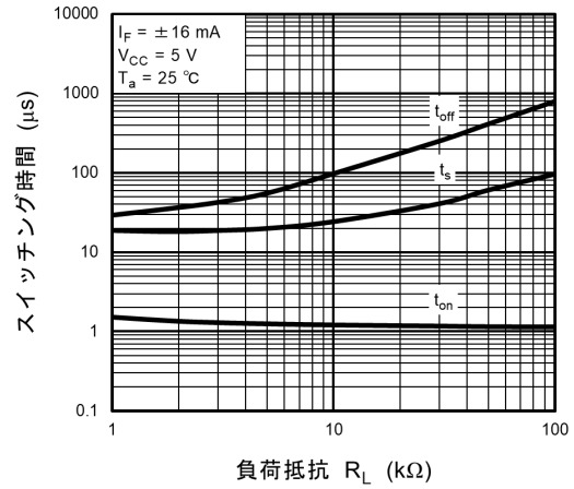
図 11.14 スwitchング時間 - R_L
