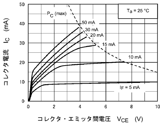
図 11.7 I_C - V_{CE}
