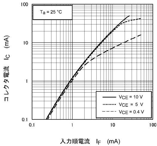
図 11.9 I_C - I_F
