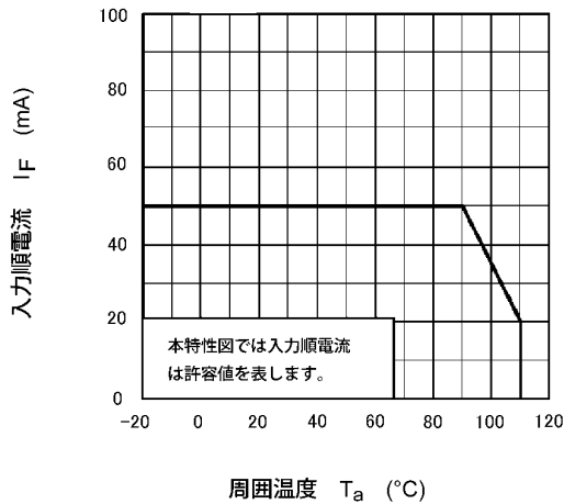
図 11.1 I_F - T_a
