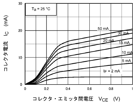
図 11.8 I_C - V_{CE}
