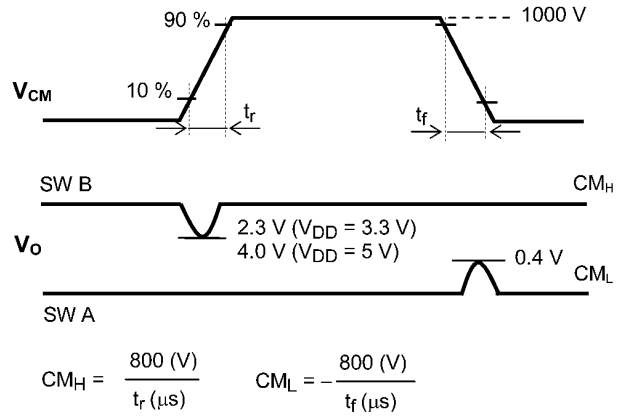
図 12.1.7 コモンモード過渡耐性測定回路, 波形
