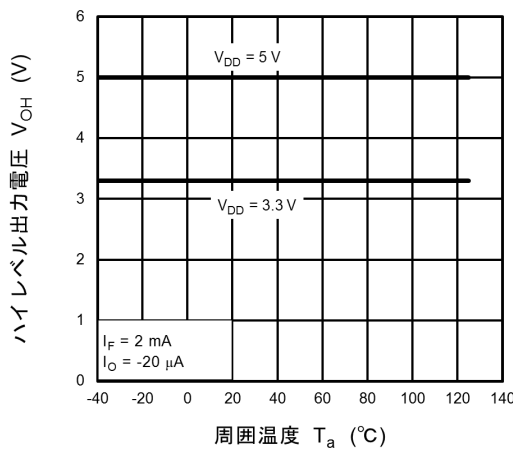
図 12.2.5 V_{OH} - T_a
