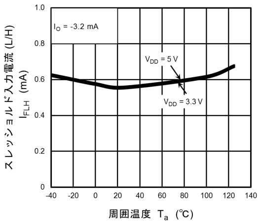
図 12.2.9 I_{FLH} - T_a
