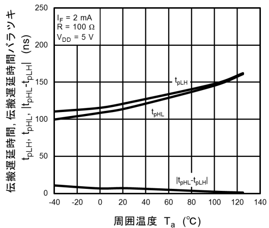
図 12.2.12 t_{pLH}, t_{pHL}, |t_{pHL} - t_{pLH}| - T_a
