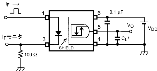
図 12.1.6 伝搬遅延時間測定回路, 波形
