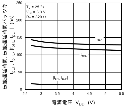
図 12.2.13 t_{pLH} , t_{pHL} , |t_{pHL} - t_{pLH}| - V_{DD}
