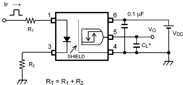
図 12.1.5 伝搬遅延時間測定回路, 波形
