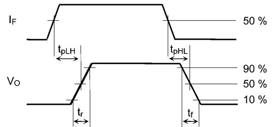
図 12.1.5 伝搬遅延時間測定回路, 波形
