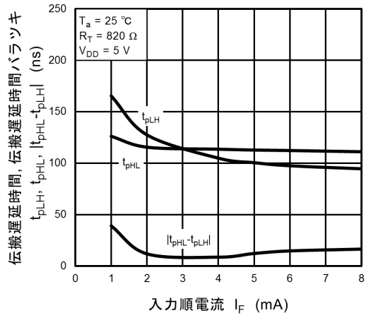
図 12.2.14 t_{pLH} , t_{pHL} , |t_{pHL} - t_{pLH}| - I_F
