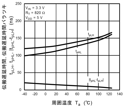
図 12.2.11 t_{pLH}, t_{pHL}, |t_{pHL} - t_{pLH}| - T_a
