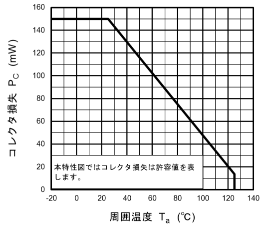
図 11.2 P_C - T_a
