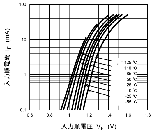
図 11.4 I_F - V_F
