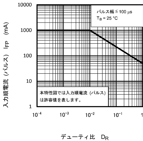
図 11.3 I_{FP} - D_R
