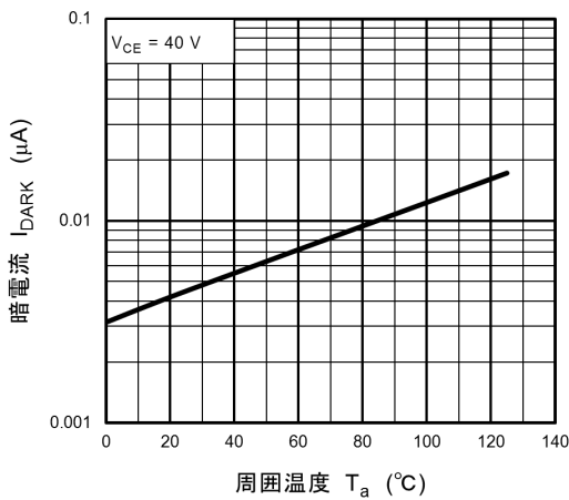
図 11.9 I_{\text{DARK}} - T_a
