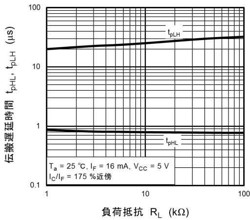
図 11.15 t_{pHL}, t_{pLH} - R_L
