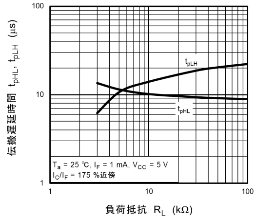
図 11.14 t_{pHL}, t_{pLH} - R_L
