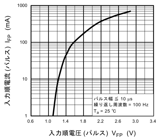
図 11.6 I_{FP} - V_{FP}
