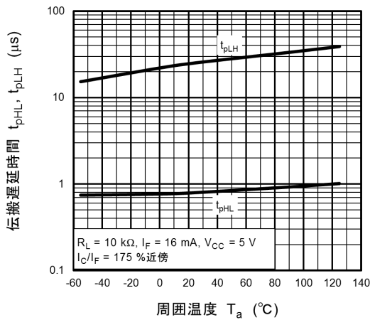
図 11.17 t_{pHL}, t_{pLH} - T_a
