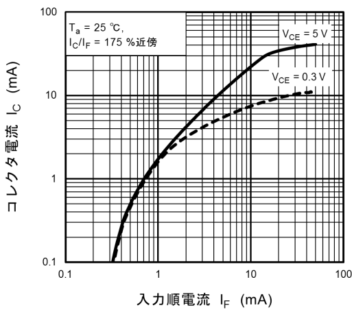
図 11.11 I_C - I_F
