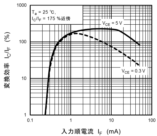
図 11.12 I_C/I_F - I_F
