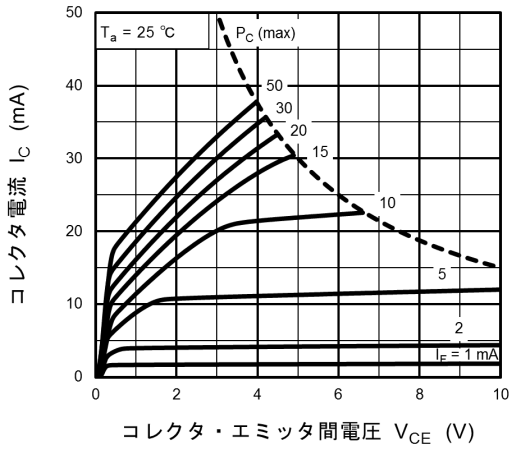
図 11.7 I_C - V_{CE}
