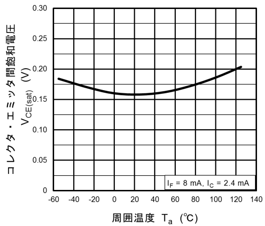
図 11.10 V_{CE(\text{sat})} - T_a
