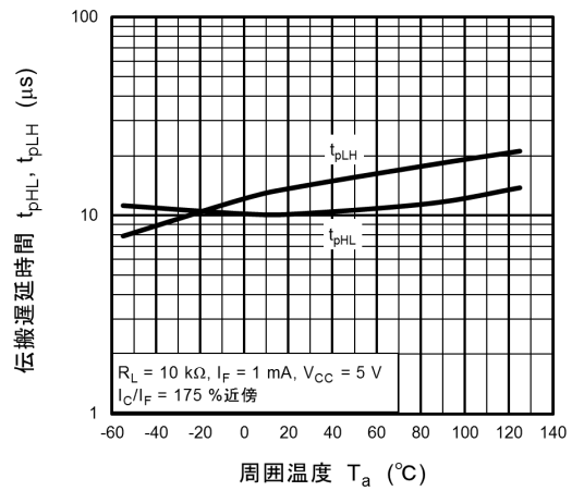
図 11.16 t_{pHL}, t_{pLH} - T_a
