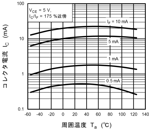
図 11.13 I_C - T_a
