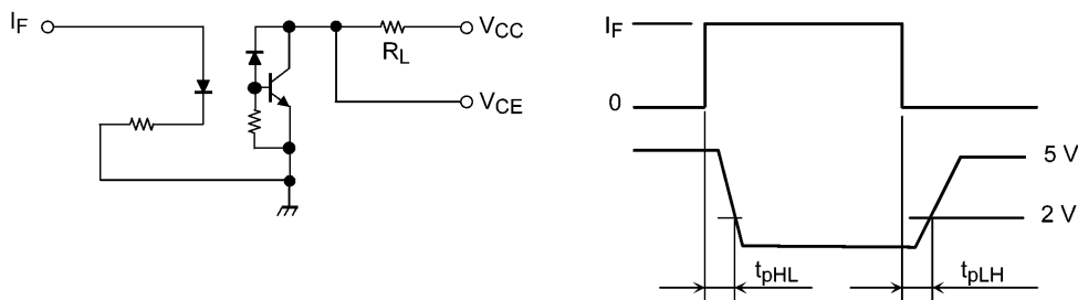
図 10.1 スイッチング時間測定回路, 波形
