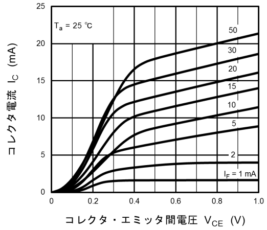
図 11.8 I_C - V_{CE}
