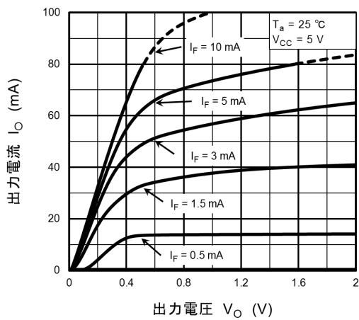
出力電流 I_O (mA) 出力電圧 V_O (V) 図 12.2.11 I_O - V_O
