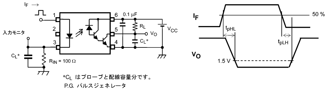
図 12.1.1 伝搬遅延時間測定回路, 波形
