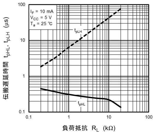
図 12.2.17 t_{pHL}, t_{pLH} - R_L
