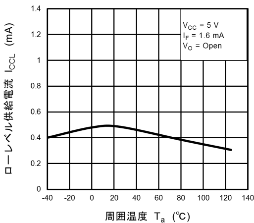
図 12.2.5 I_{CCL} - T_a
