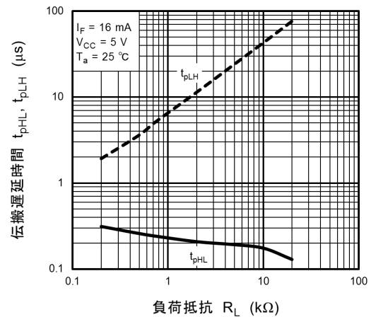
図 12.2.18 t_{pHL}, t_{pLH} - R_L
