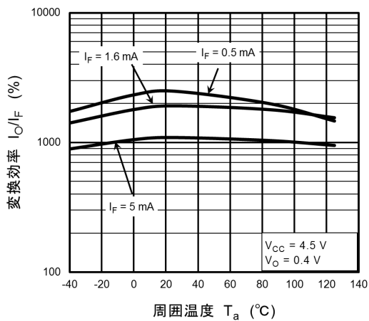
変換効率 I_O/I_F (%) 周囲温度 T_a (°C) 図 12.2.9 I_O/I_F - T_a
