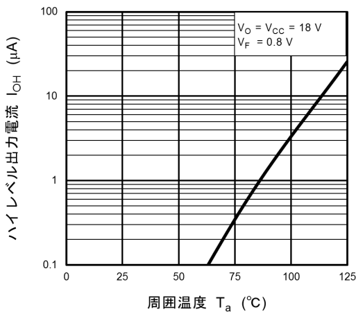
図 12.2.3 I_{OH} - T_a
