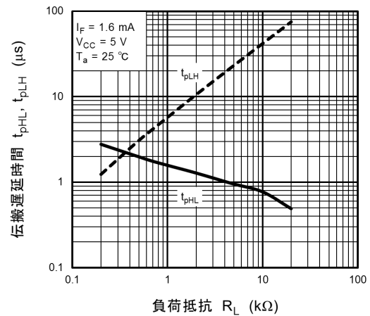
図 12.2.16 t_{pHL}, t_{pLH} - R_L
