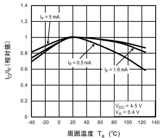
I_O/I_F (相対値) 周囲温度 T_a (°C) 図 12.2.10 I_O/I_F - T_a
