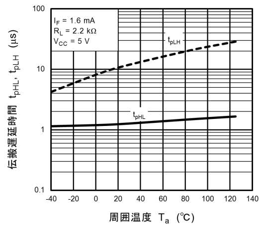
伝搬遅延時間 t_{pHL}, t_{pLH} ( \mu s ) 周囲温度 T_a (°C) 図 12.2.12 t_{pHL}, t_{pLH} - T_a
