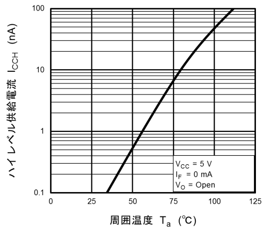
図 12.2.4 I_{CCH} - T_a
