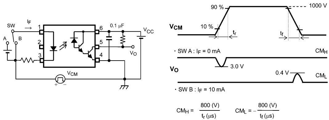
図 12.1.2 コモンモード過渡耐性測定回路, 波形
