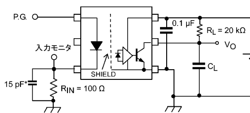
図 13.1.6 伝搬遅延時間測定回路, 波形
