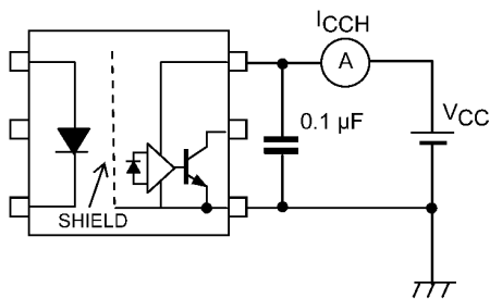
図 13.1.3 I CCH 測定回路
