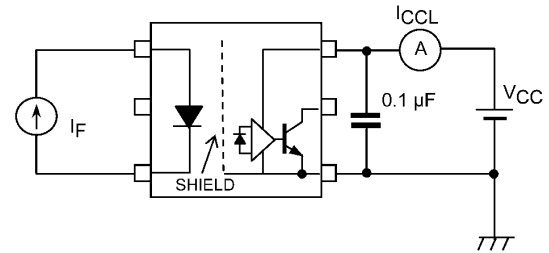
図 13.1.4 I CCL 測定回路
