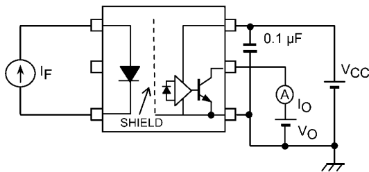
図 13.1.5 I O 測定回路
