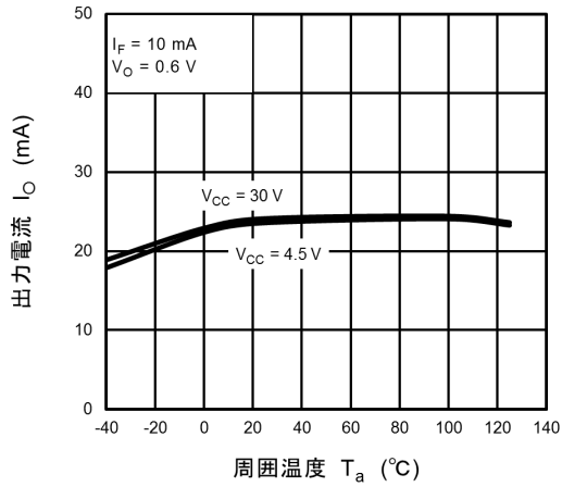
図 13.2.7 I_O - T_a
