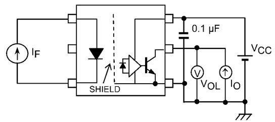
図 13.1.2 V OL 測定回路
