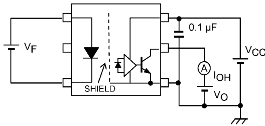
図 13.1.1 I OH 測定回路
