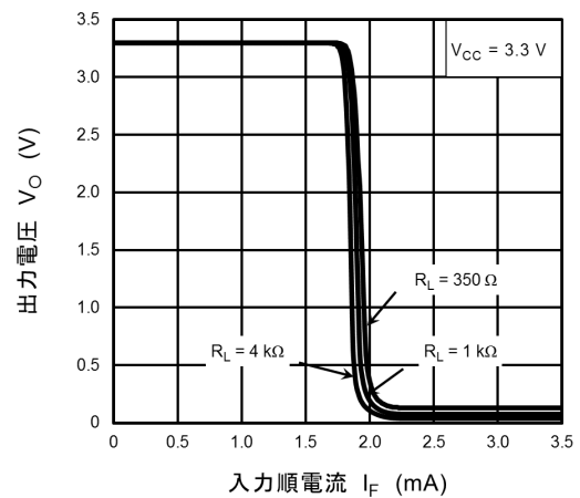
図 13.2.6 V_O - I_F
