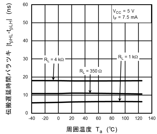
図 13.2.12 |t_{pHL} - t_{pLH}| - T_a
