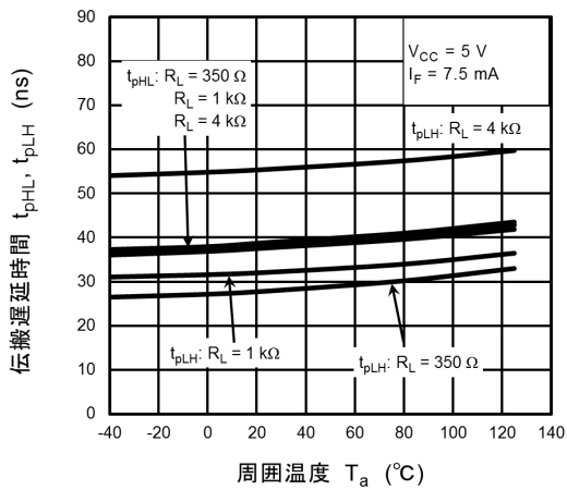
図 13.2.11 t_{pHL}, t_{pLH} - T_a
