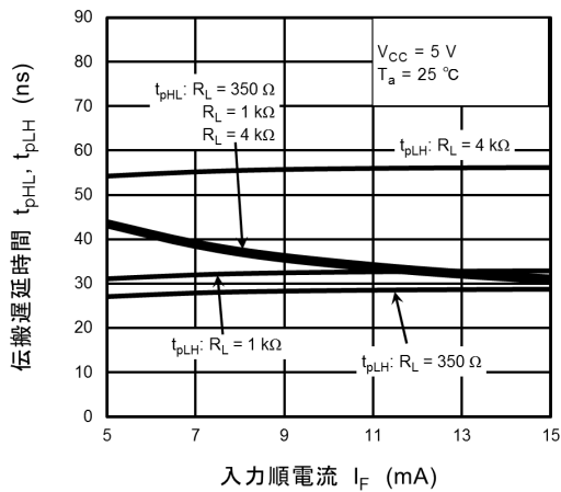
図 13.2.15 t_{pHL} , t_{pLH} - I_F
