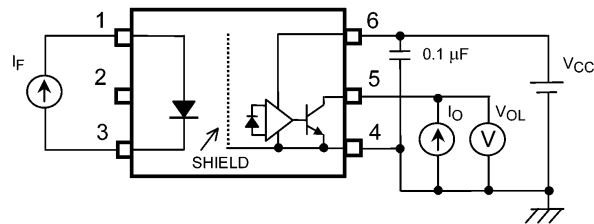
図 13.1.2 V OL 測定回路
