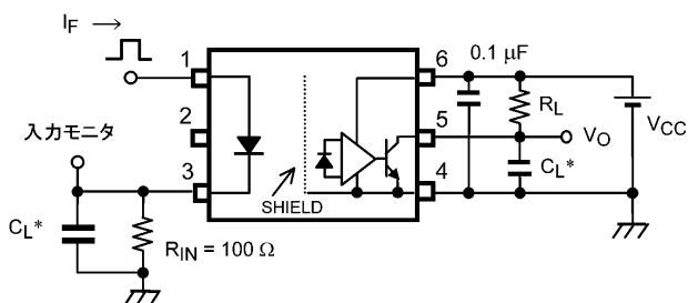
図 13.1.5 伝搬遅延時間測定回路, 波形
