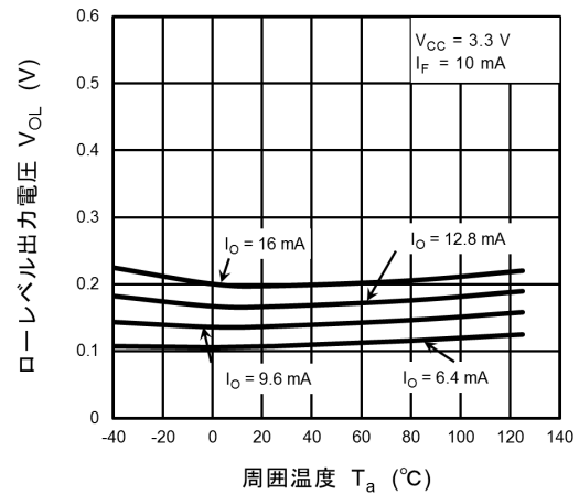
図 13.2.4 V_{OL} - T_a
