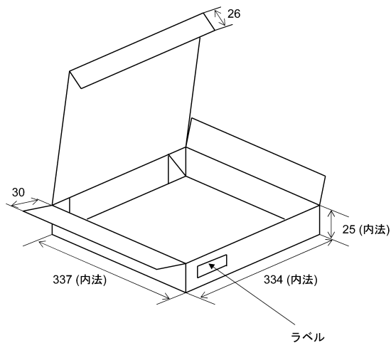
図 18.4.1 1リール入り梱包箱 (unit: mm)
