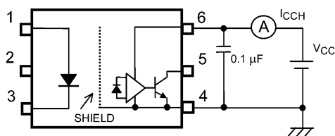
図 13.1.3 I CCH 測定回路
