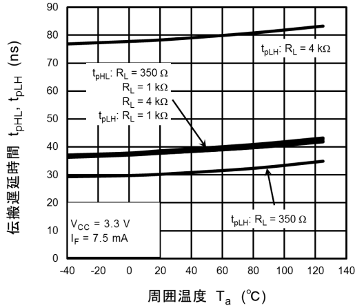
図 13.2.13 t_{pHL} , t_{pLH} - T_a
