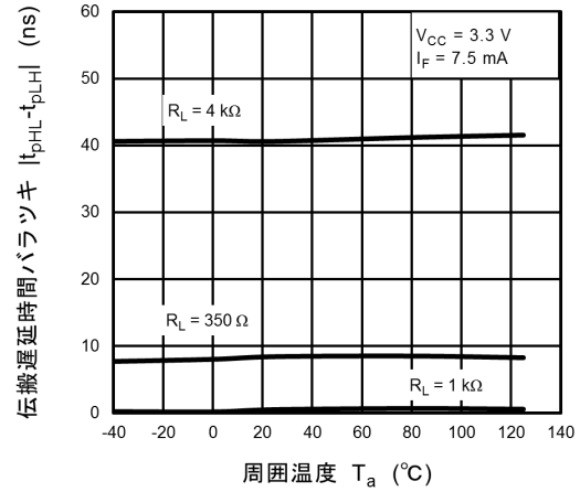
図 13.2.14 |t_{pHL} - t_{pLH}| - T_a
