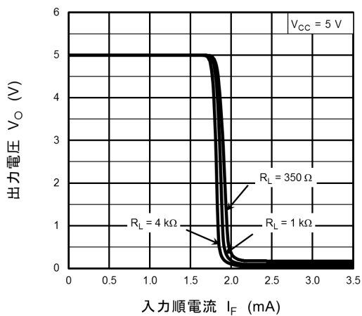
図 13.2.5 V_O - I_F
