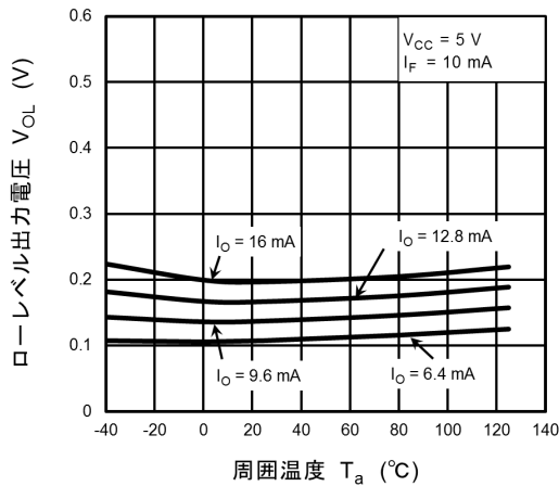
図 13.2.3 V_{OL} - T_a
