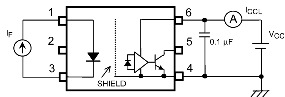
図 13.1.4 I CCL 測定回路
