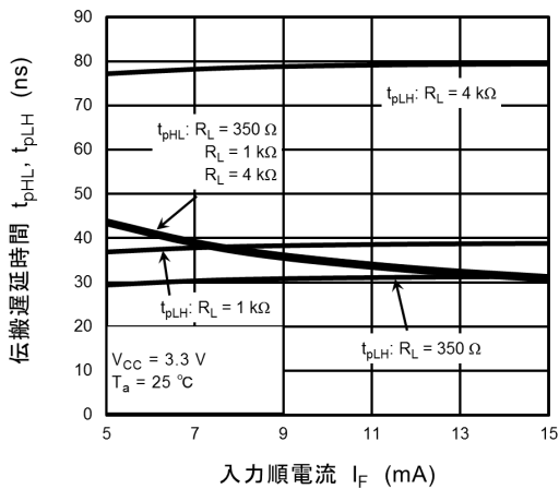
図 13.2.17 t_{pHL} , t_{pLH} - I_F
