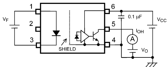
図 13.1.1 I OH 測定回路
