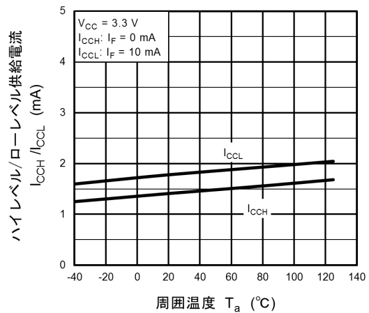
図 13.2.10 I_{CCH}, I_{CCL} - T_a
