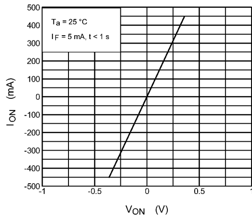
図 12.4 I_{ON} - V_{ON}
