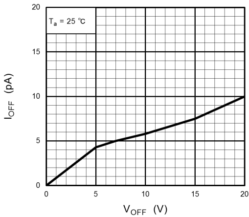
図 12.9 I_{OFF} - V_{OFF}
